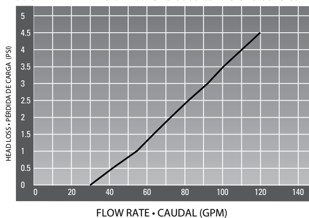
D.E. FILTER • FILTRO DE T.I. - 570-0060-09LE & 570-0048-09LE
